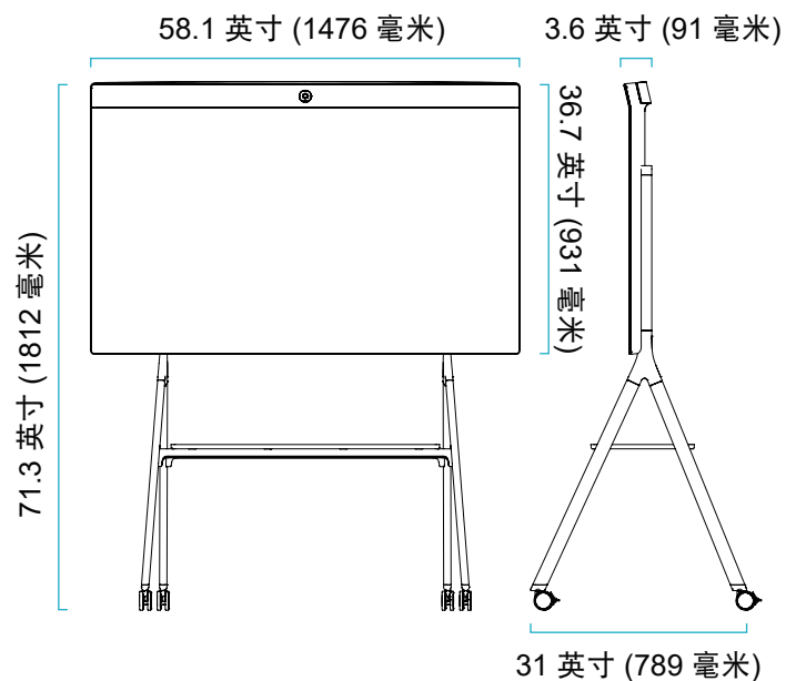
Neat Board 触屏式视讯会议终端 (含落地支架) 重量: 124.6 磅 (56.5 千克)
