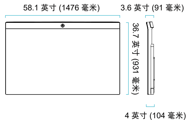
Neat Board 触屏式视讯会议终端 (含壁挂支架) 重量: 111.6 磅 (50.6 千克)
